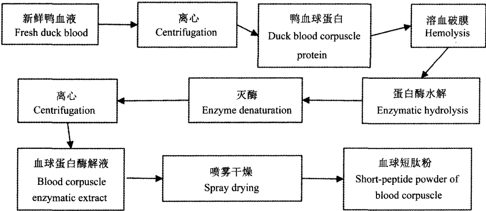
图 1 酶法水解鸭血球蛋白工艺流程
